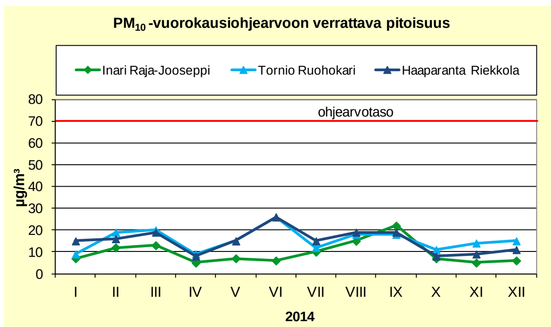
Kuva 23. Hengitettävien hiukkasten vuorokausiohjearvoon verrattavia pitoisuuksia Tornion Ruohokarissa ja Haaparannan Riekkolassa sekä Inarin Raja-Joosepin taustasemalla vuonna 2014.
