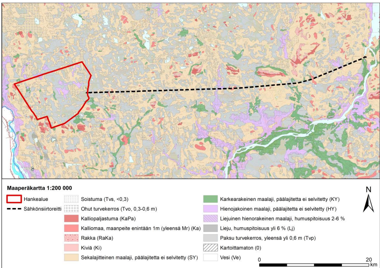
Kuva 5.20. Kaava-alueen ja sähkönsiirtoreitin maaperä (GTK Maaperäkartta 1:200 000).
