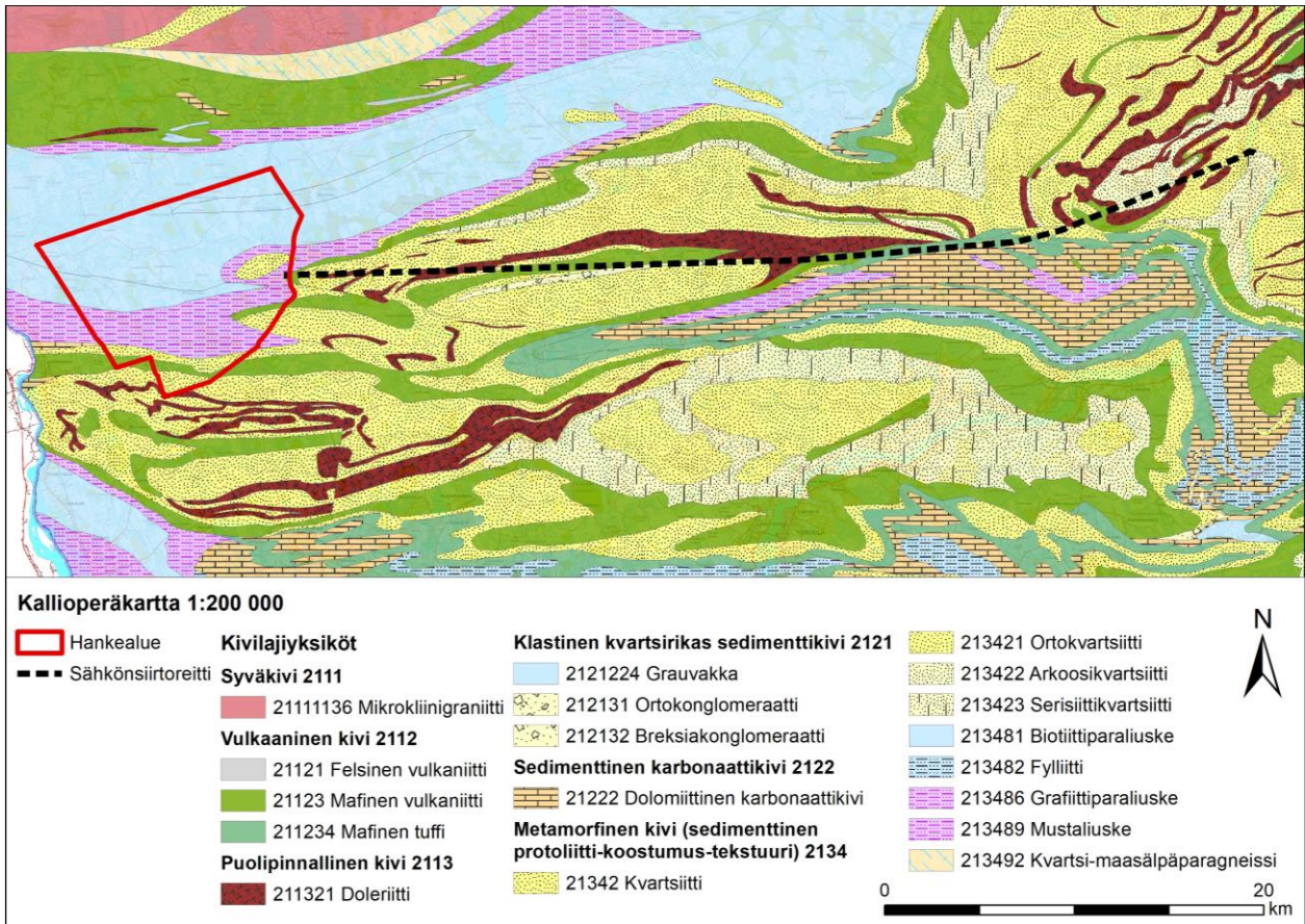
Kuva 5.19. Kaava-alueen ja sähkönsiirtoreitin kallioperä (GTK Kallioperäkartta 1:200 000).
