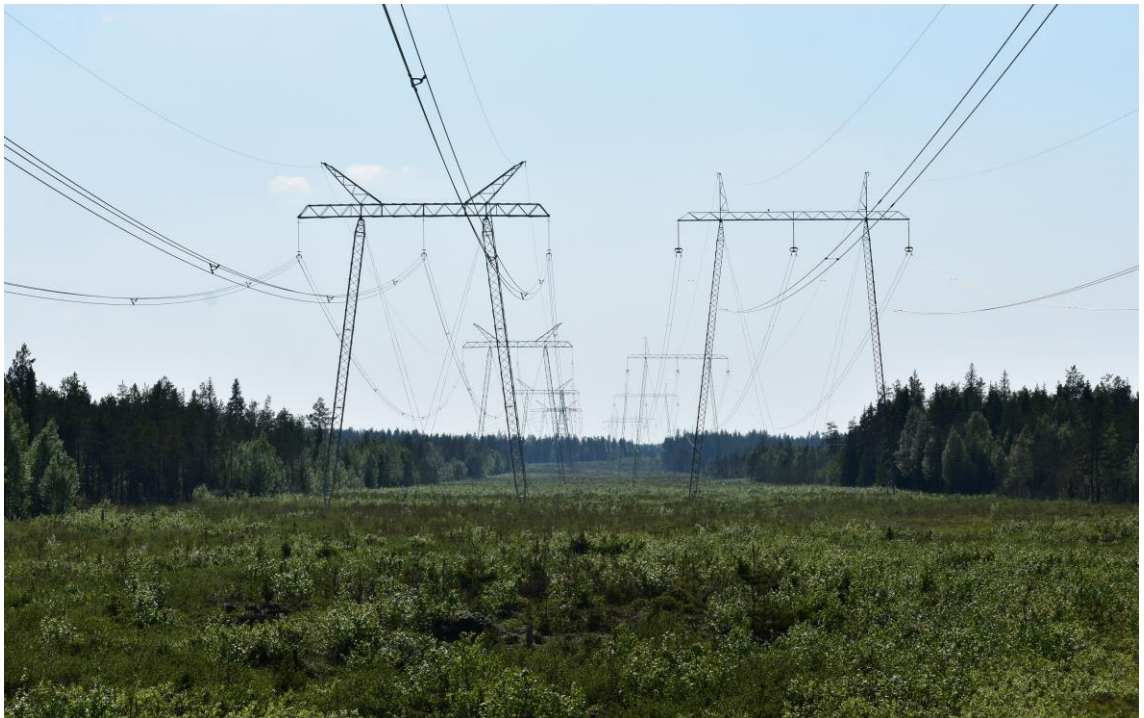
Kuva 5.28. Hankkeen sähkönsiirtoreittiä on tutkittu levennettävän 33 metriä voimajohtokäytävän osalta. Reitin itäosassa johtokäytävässä on rinnakkain kaksi 400 kV voimajohtoa.
