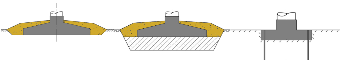
Kuva 2.12. Tuulivoimalat voidaan perustaa useilla eri tavoilla. Periaatekuvat maavaraisesta teräsbetoniperustuksesta, teräsbetoniperustuksesta massanvaihdon kanssa sekä kallioankkuroidulla teräsbetoniperustuksesta.
