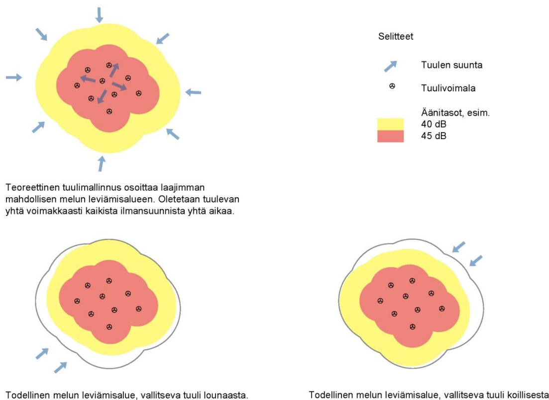
Kuva 4.8. Mallikuva teoreettisesta melumallinnuksesta ylhäällä ja todellisen tilanteen mukaisesta tuulivoimamelun leviämisestä alarivissä.
