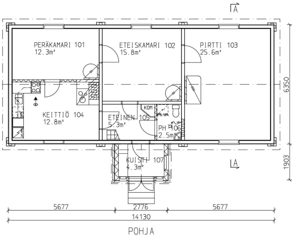
Kuva 1 Viippolan ensimmäisen kerroksen pohjakaava.
