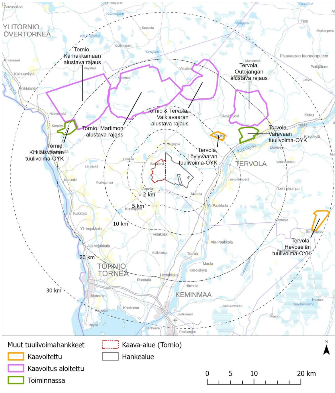
Kuva 5.4. Kaava- ja hankealue suhteessa lähiseudun (noin 30 kilometrin säde) tuulivoimahankkeisiin (22.8.2022).
