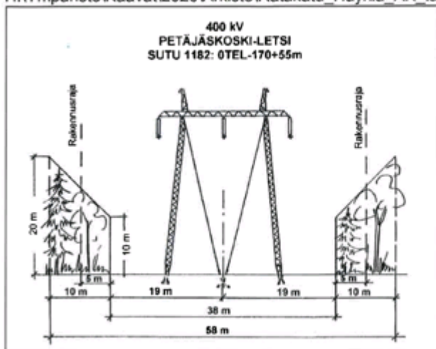
Kuva 2. Fingridin 400 kV voimajohdon Petäjäsken - Letsi poikkileikkaus.
