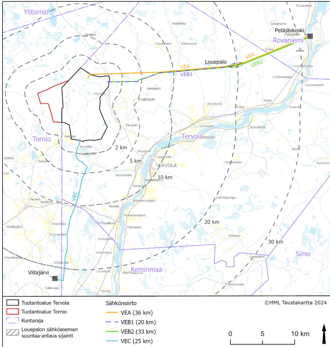
Kuva 2.3. Sähkönsiirron vaihtoehdot.
